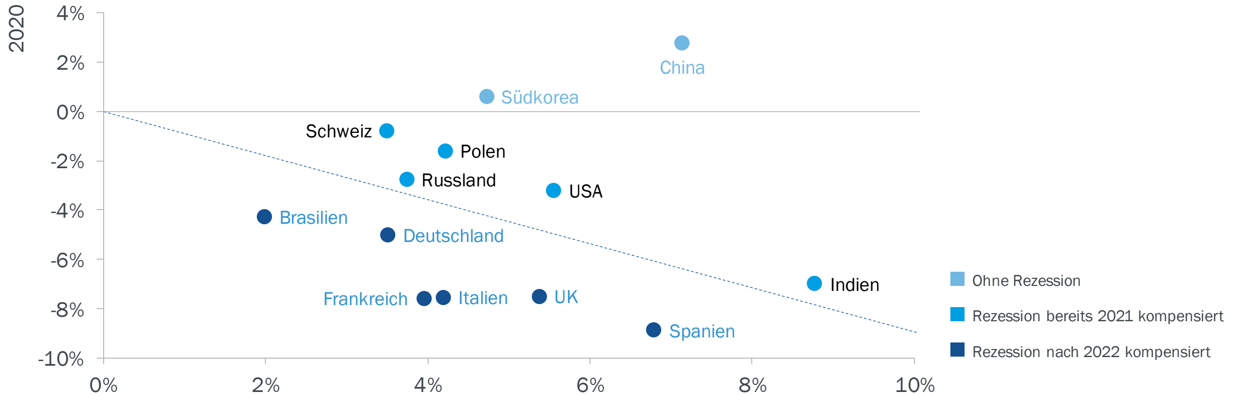
Veränderung des BIP in ausgewählten Ländern, 2020 und 2021
